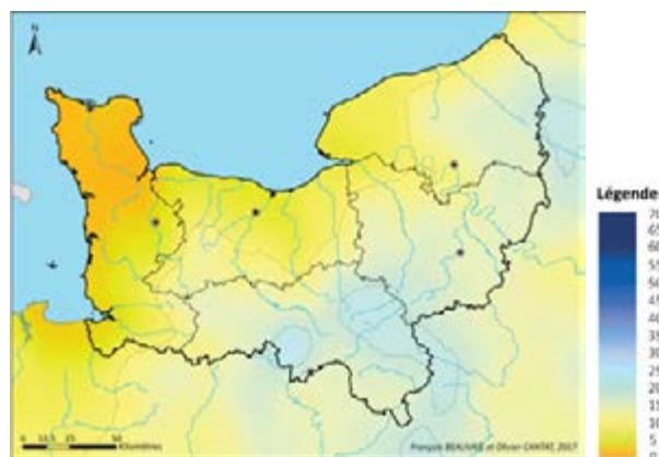
FIGURE 17. SCENARIOS CONCERNANT L'ÉVOLUTION DU NOMBRE DE JOURS DE GEL RCP 2.6 (AVEC POLITIQUE CLIMATIQUE - DROITE) ET RCP 8.5 (SANS POLITIQUE CLIMATIQUE - GAUCHE) À L'HORIZON 2100
