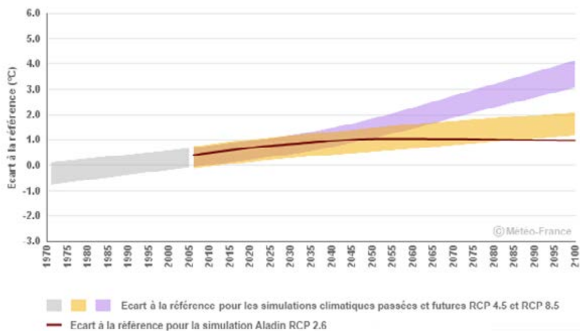
FIGURE 6. ÉVOLUTION DES TEMPÉRATURES MOYENNES ANNUELLES EN BASSE NORMANDIE SELON LES TROIS SCÉNARIIS D'ÉVOLUTION, 1959-2017 Source : Météo France
