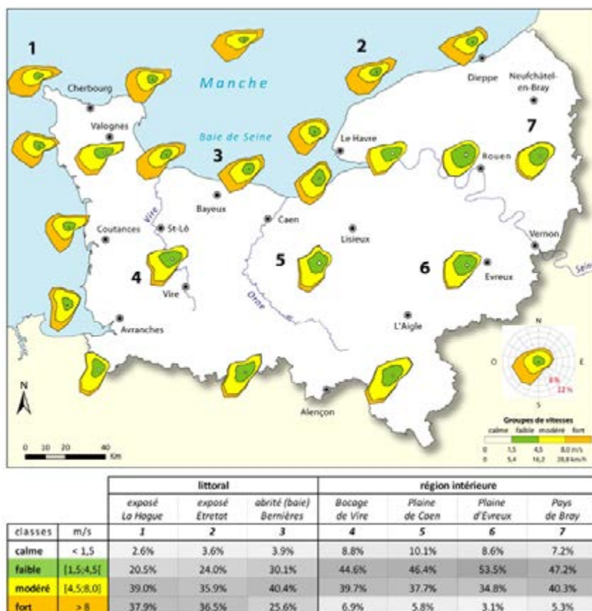
FIGURE 14. CARTE ET TABLEAU DE SYNTHÈSE ÉTABLIS À PARTIR DES VENTS TRI-HORAIRES MODÉLISÉS À PARTIR D'ALADIN (MÉTÉO FRANCE), 1999-2000
