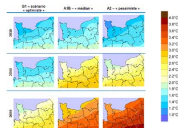
FIGURE 9. TEMPÉRATURES MOYENNES ESTIVALES AUX HORIZONS 2030-2050-2080 (ÉCART À LA RÉFÉRENCE EN DEGRÉ) Source : Météo France, DATAR 2011
