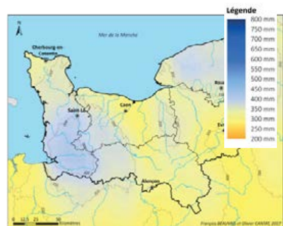
FIGURE 12. CUMUL MOYEN DE PRÉCIPITATIONS ENTRE OCTOBRE ET MARS (GAUCHE) ET ENTRE AVRIL ET SEPTEMBRE (DROITE), 1976-2005
