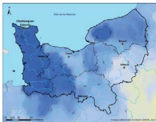
FIGURE 12. CUMUL MOYEN DE PRÉCIPITATIONS ENTRE OCTOBRE ET MARS (GAUCHE) ET ENTRE AVRIL ET SEPTEMBRE (DROITE), 1976-2005
